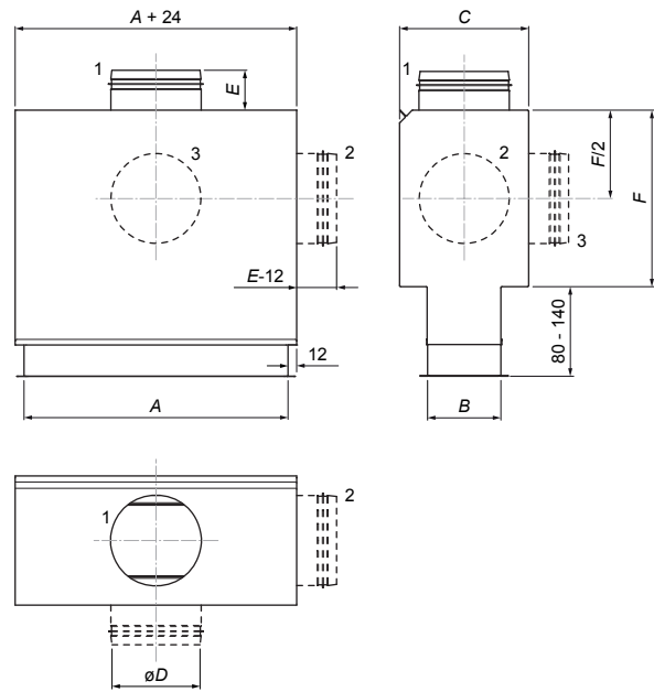
Obr. : Základné rozmery pretlakovej komory ODEN
